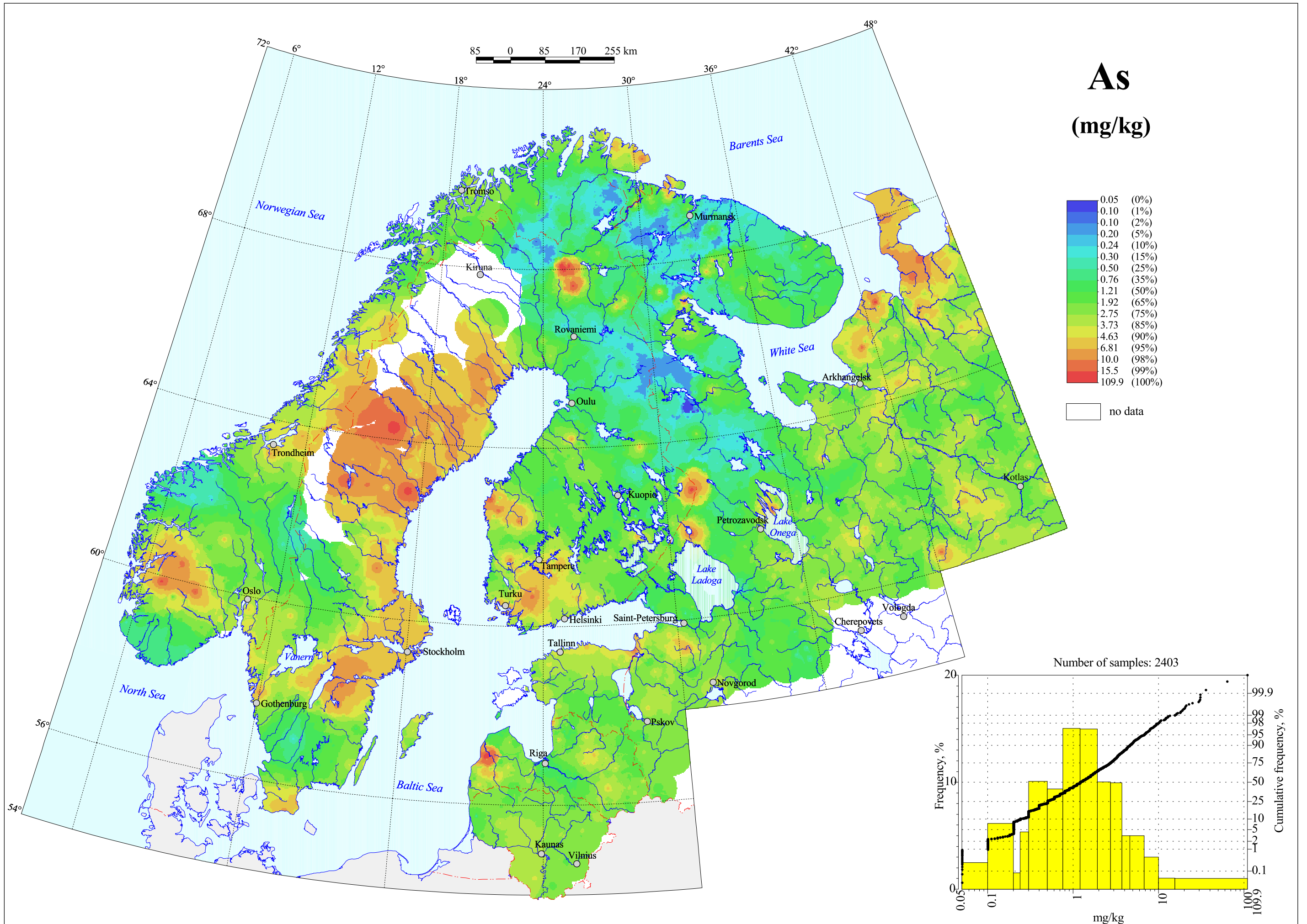
Arsenic in C-horizon, Grain Size <2 mm, Aqua regia Extraction
